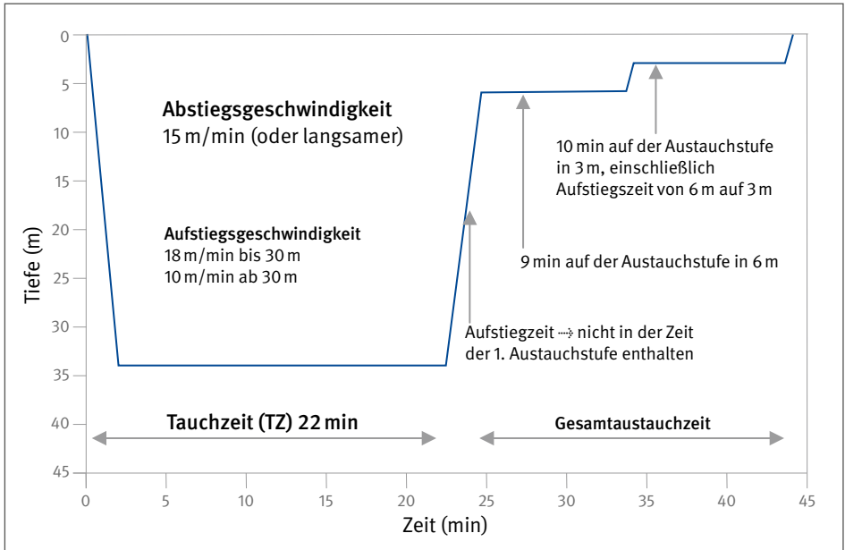
Abb. 2 Definitionen zum Beispiel 2 (Tauchgangsberechnung mit Atemluft)
