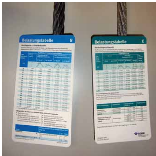
Bild 8-1: Die Belastungstabelle gibt für das schmiegsame Kabelschlagseil (rechts) eine geringere Tragfähigkeit an als für die links dargestellten Litzenseile
