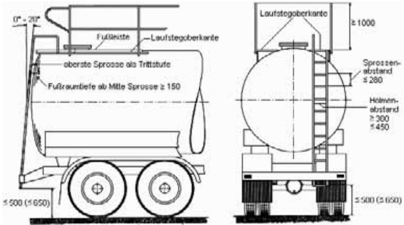
Fußraumtiefe
