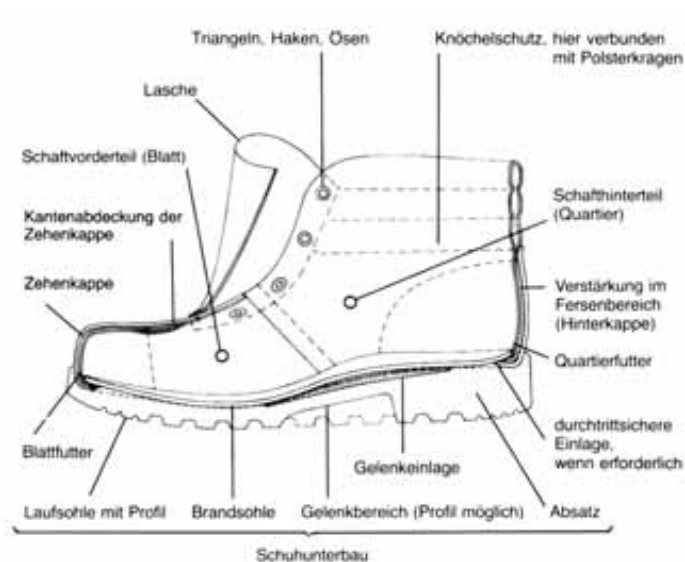
Bild 1: Beispiele für Bestandteile eines Schuher
