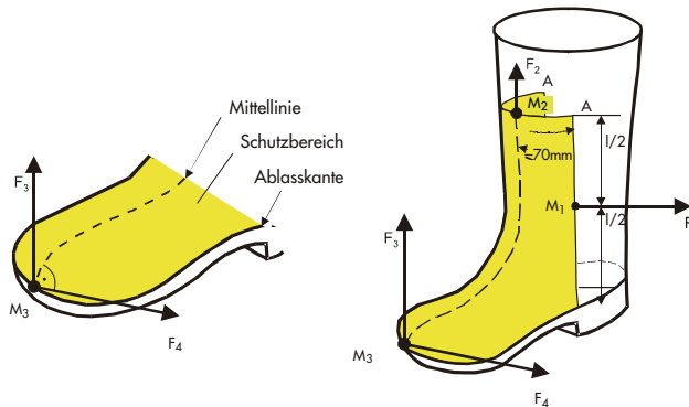
Bild 10 Gamasche mit Mindestschutzbereich
