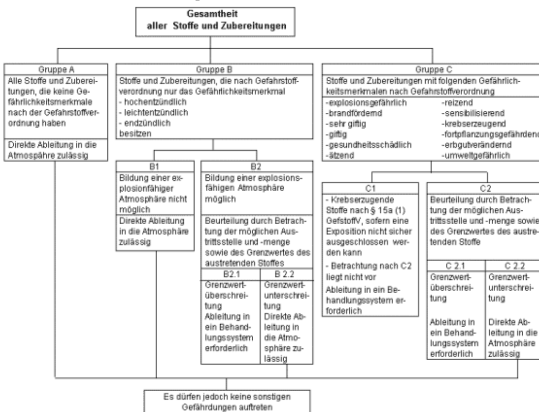
Bild 1 Abschnitt 3.4.1 Schema des gefahrlosen Ableitens nach Gefahrstoffmerkmalen
